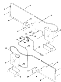
ETB-011808, Znacznik pianowy bez sprężarki
