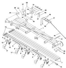
ETB-011781, Wysięgnik hydr. 16 m prawy (1/2)
