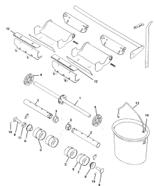
ETB-011826, Wałek dozujący mikrogranulatu prawy -pojedynczy
