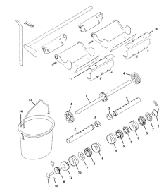
ETB-011817, Wałek dozujący mikrogranulatu lewy -nawóz 15 m-
