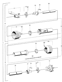
ETB-011789, Wałek przekątnikowy ze sprzęgłem ciernym -710 mm-
