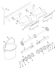
ETB-011819, Wałek dozujący mikrogranulatu lewy - podwójny 15 m
