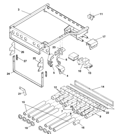
ETB-011804, Śluza iniektora 18 m lewa
