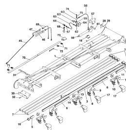
ETB-011783, Wysięgnik hydr. 18 m lewy (1/2)
