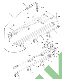
ETB-011771, Wysięgnik 10 m lewy
