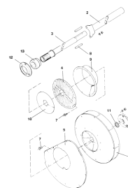
ETB-011791, Koło łopatkowe
