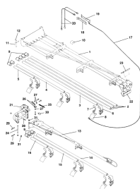
ETB-011774, Wysięgnik 12 m prawy
