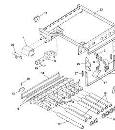
ETB-011801, Śluza iniektora 12 m prawa
