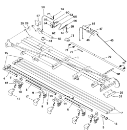
ETB-011785, Wysięgnik hydr. 18 m prawy (1/2)
