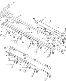
ETB-011786, Wysięgnik hydr. 18 m prawy (2/2)
