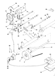
ETB-011788, Napęd, wersja H
