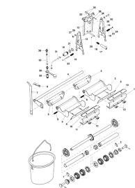
ETB-011792, Urządzenie podstawowe F lewe
