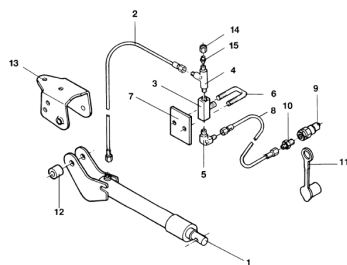
ETB-011814, Sterowanie hydr. belki polowej prawe
