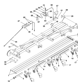
ETB-011779, Wysięgnik hydr. 16 m lewy (1/2)
