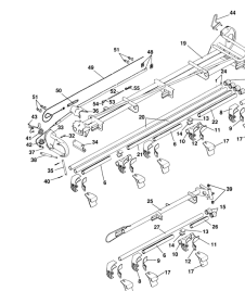
ETB-011776, Wysięgnik hydr. 15 m lewy (2/2)
