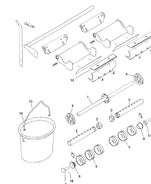
ETB-011821, Wałek dozujący mikrogranulatu lewy -podwójny 10, 12, 16, 18 m-
