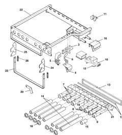
ETB-011802, Śluza iniektora 15 m + 16 m lewa
