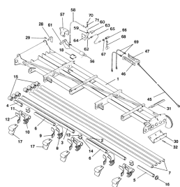
ETB-011777, Wysięgnik hydr. 15 m prawy (1/2)
