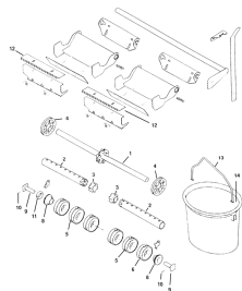
ETB-011818, Wałek dozujący mikrogranulatu prawy - podwójny 15 m
