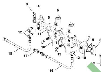
ETB-011811, Blok zaworów elektromagnetycznych -dwukrotny-
