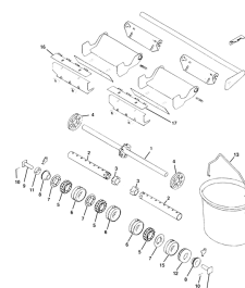
ETB-011816, Wałek dozujący mikrogranulatu prawy -nawóz 15 m-
