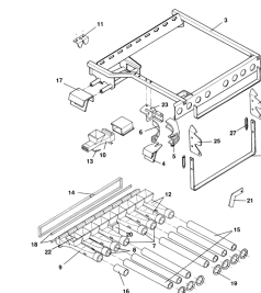
ETB-011805, Śluza iniektora 18 m prawa
