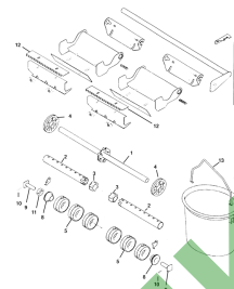
ETB-011820, Wałek dozujący mikrogranulatu prawy -podwójny 10, 12, 16, 18 m-
