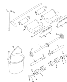
ETB-011825, Wałek dozujący mikrogranulatu lewy -pojedynczy 10, 12, 16, 18 m-
