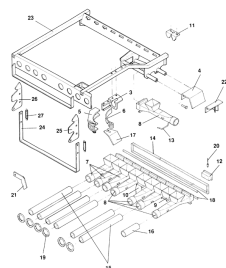
ETB-011798, Śluza iniektora 10 m lewa
