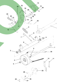
ETB-011787, Napęd, wersja F
