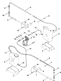
ETB-011807, Znacznik pianowy ze sprężarką
