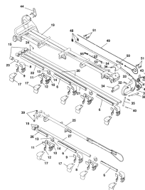
ETB-011782, Wysięgnik hydr. 16 m prawy (2/2)
