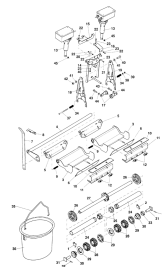
ETB-011795, Urządzenie podstawowe H lewe
