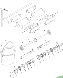
ETB-011823, Wałek dozujący mikrogranulatu lewy -nawóz 10, 12, 16, 18 m-
