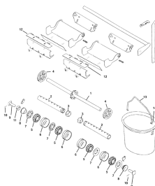
ETB-011822, Wałek dozujący mikrogranulatu prawy -nawóz 10, 12, 16, 18 m-
