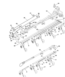
ETB-011780, Wysięgnik hydr. 16 m lewy (2/2)
