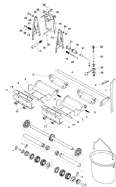
ETB-011794, Urządzenie podstawowe F prawe
